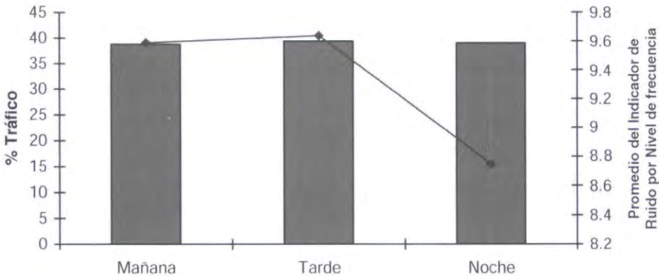
Figura N° 3. Comparación del por ciento de Tráfico y promedio del Indicador de Ruido por Subcanal de Frecuencia cuando se generó tráfico en el horario de la noche.
