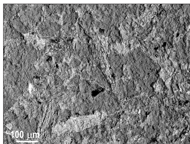
Obr. 3: BSE obraz siltové břidlice (vzorek M1276) z velkolomu Mokrá.
