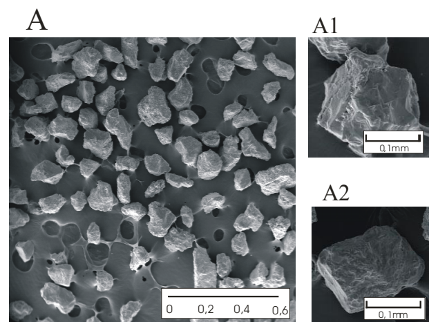
Obr. 2 – křemenná zrna z lokality Hybešova – miocenní sedimenty (téggl), A1 – celkový pohled, A1 – ostrohranná zrna s polozaoblennými hranami, A2 – polozaoblenná zrna postížená postsedimentárními procesy rozpouštění. Fig. 2 – quartz grains from the Hybešova locality – Miocene sediments (téggl), A – whole view, A1 – angular grains with subrounded edges, A2 – subrounded grains with postsedimentary processes of dissolving.
