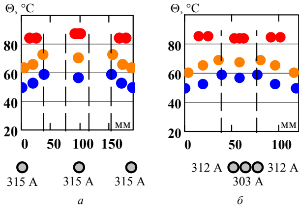
Рис. 3. Результати вимірювання температури при нагріванні трьох однофазних одножилних кабелів АПвЭгаПу 1×70/16–35 при розташуванні в горизонтальній площині на відстані одного діаметра (а) і впритул (б) з однаковим напрямком струму (схема розташування кабелів і термодар див. на рис. 1): верхні точки – температура жил; нижні точки – температура на поверхні кабелів; середні точки – температура в мідних екранах
