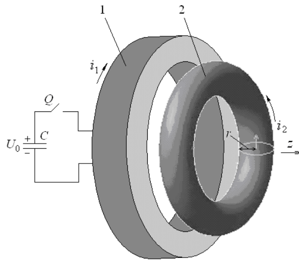
Рис. 1. Схема електродинамічного прискорювача: 1 – індуктор; 2 – струмопровідне плазмове кільце
