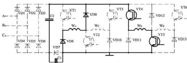
Рис. 3. Конфигурация схемы УВРД при ОКФ
