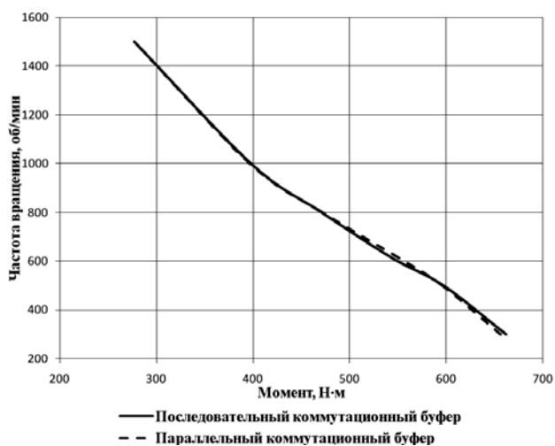
Рис. 6. Механические характеристики УВРД 2 при трехфазном питании
