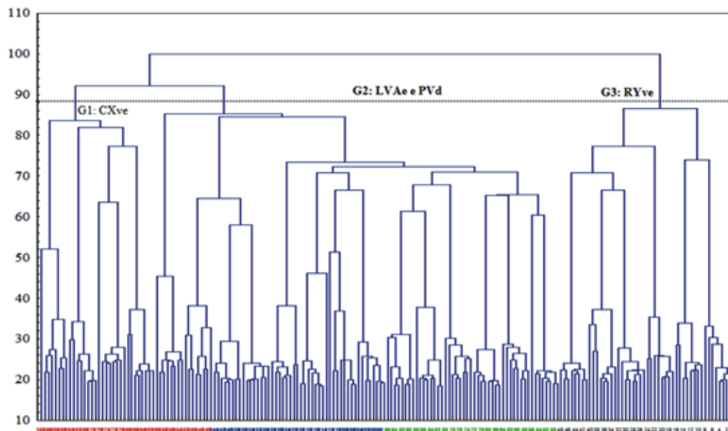
Figura 2. Dendrograma das interrelações dos solos estudados, referente ao conjunto de variáveis químicas (pH, Cl, HCO 3 CE, Ca 2+ , Mg 2+ , Na + , K + ) do segundo cultivo, pela distância euclidiana média
