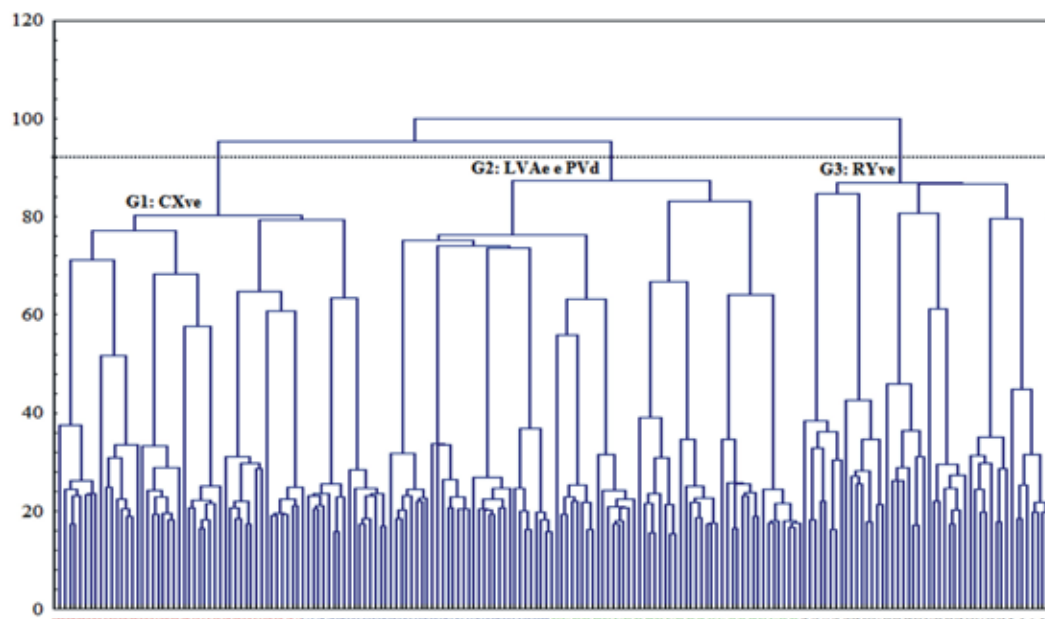
Figura 1. Dendrograma das interrelações dos solos estudados e lixiviados, referente ao conjunto de variáveis químicas (pH, CE, Ca 2+ , Mg 2+ , Na + , K + , Cl - , HCO 3 - ) do primeiro cultivo, pela distância euclidiana média
