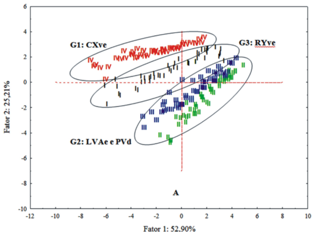
Figura 3. Análise multivariada de componentes principais para as variáveis químicas: A (primeiro cultivo) - pH, CE, Ca 2+ , Mg 2+ , Na + , K + , Cl - , HCO 3 - e B (segundo cultivo) - pH, CE, Ca 2+ , Mg 2+ , Na + , K +
