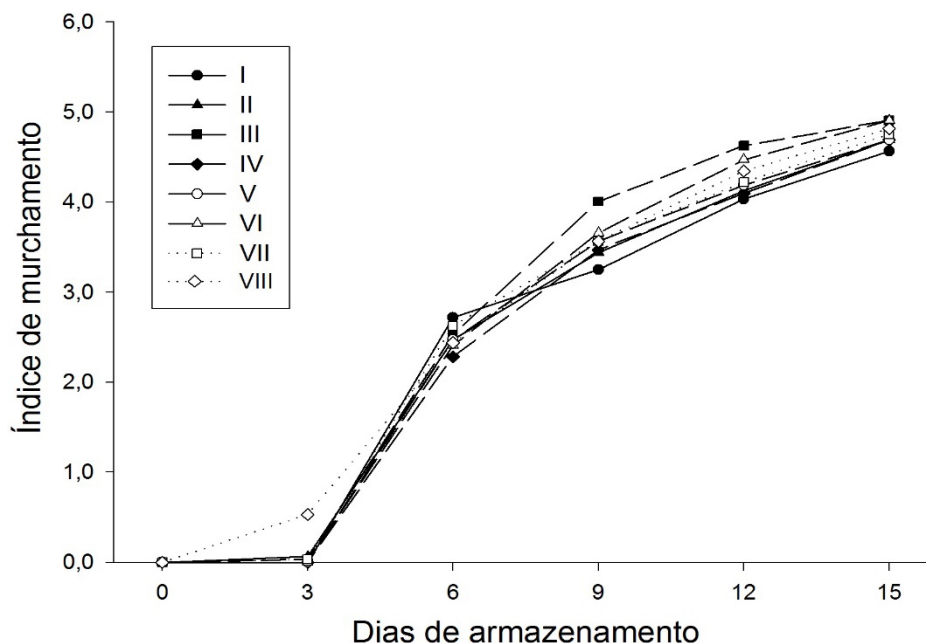
Figura 1 - Índice de murchamento de frutos de maracujá-amarelo tratados com derivados de capim-limão
