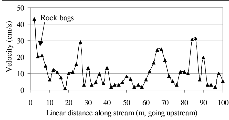
Fig. 13. Thalweg velocity
