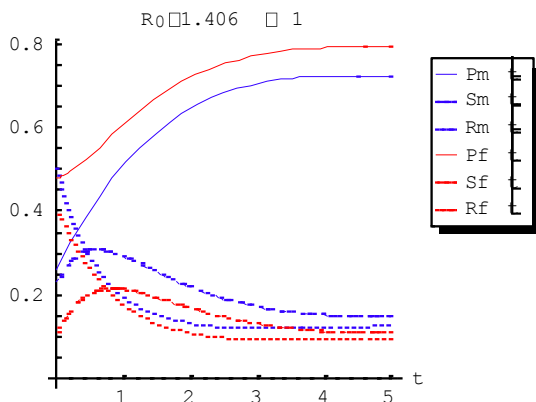
Gambar 3. Grafik Solusi dengan Nilai Awal Pm(0) = 0.26 , Sm(0) = 0.51 ,
