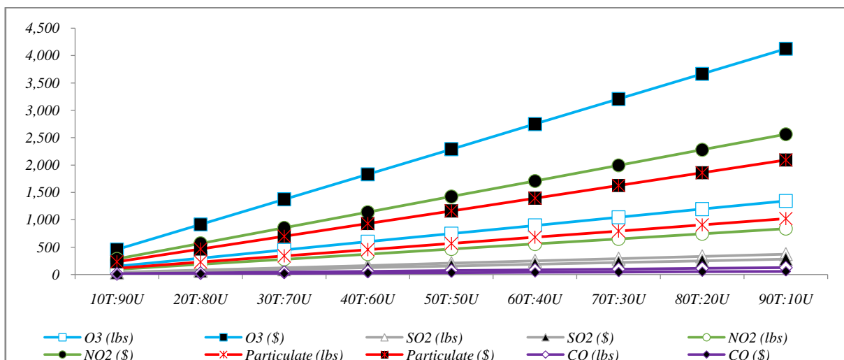
Gambar 2. Diagram garis potensi penyerapan polutan oleh canopy pohon pada berbagai skenario proporsi antar luas canopy pohon/tree (T) dan luas Urban landuse (U)
