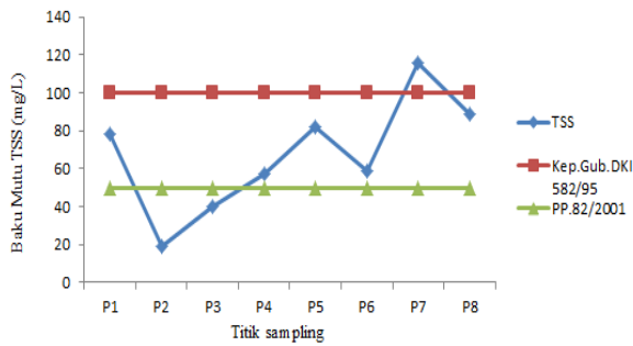
Gambar 2. Nilai TSS air Sungai Pesanggrahan
