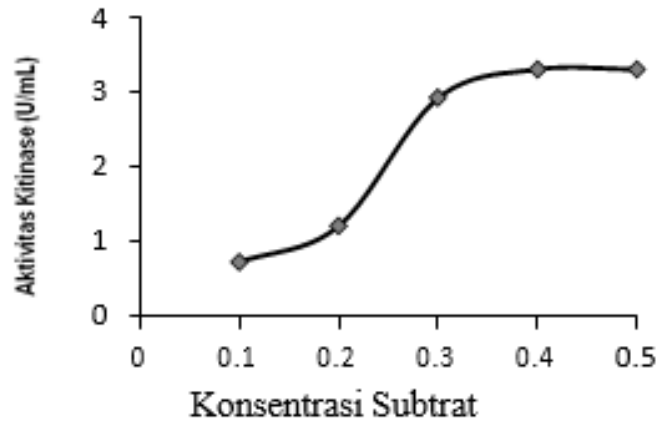
Gambar 6. Pengaruh konsentrasi substrat terhadap aktivitas kitinase pada kondisi pH 6 dan suhu 35°C
