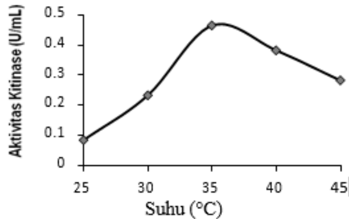
Gambar 5. Pengaruh suhu terhadap aktivitas kitinase pada pH 6
