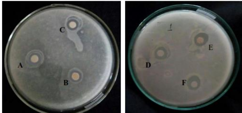
Gambar 2. Zona bening produksi aktivitas kitinase isolat IK A
