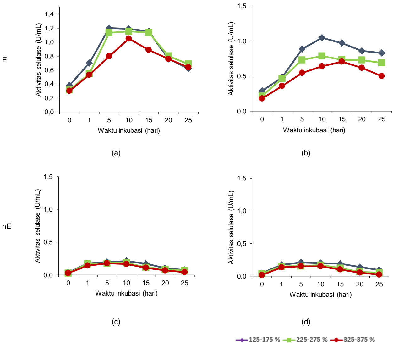
Gambar 2 Aktivitas Selulase pada tiga kadar air dalam a) Gambut steril dengan pemberian selulase, b) Gambut non-steril dengan pemberian selulase, c) Gambut steril tanpa pemberian selulase, dan d) Gambut non-steril tanpa pemberian selulase.
