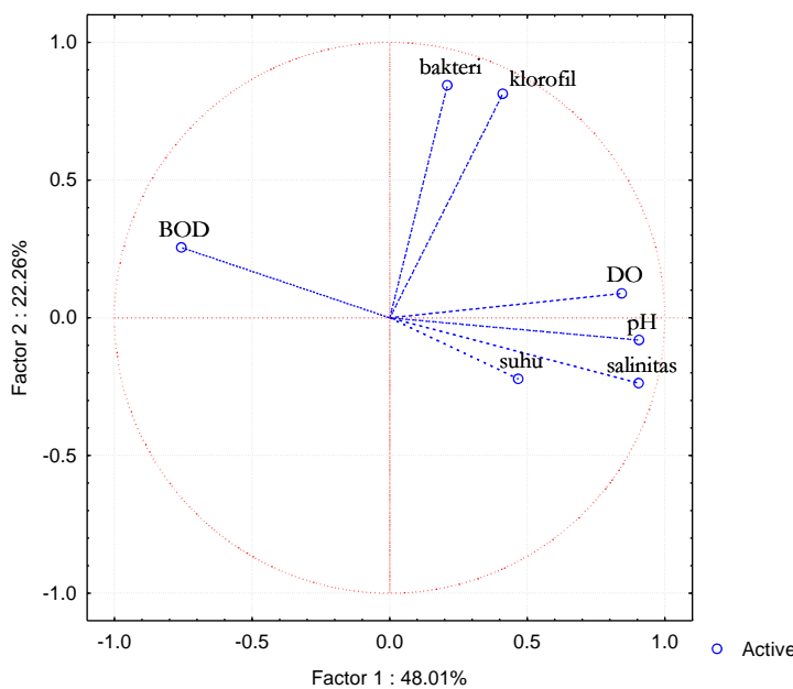
Gambar 6 Biplot PCA hubungan antar parameter penelitian.
