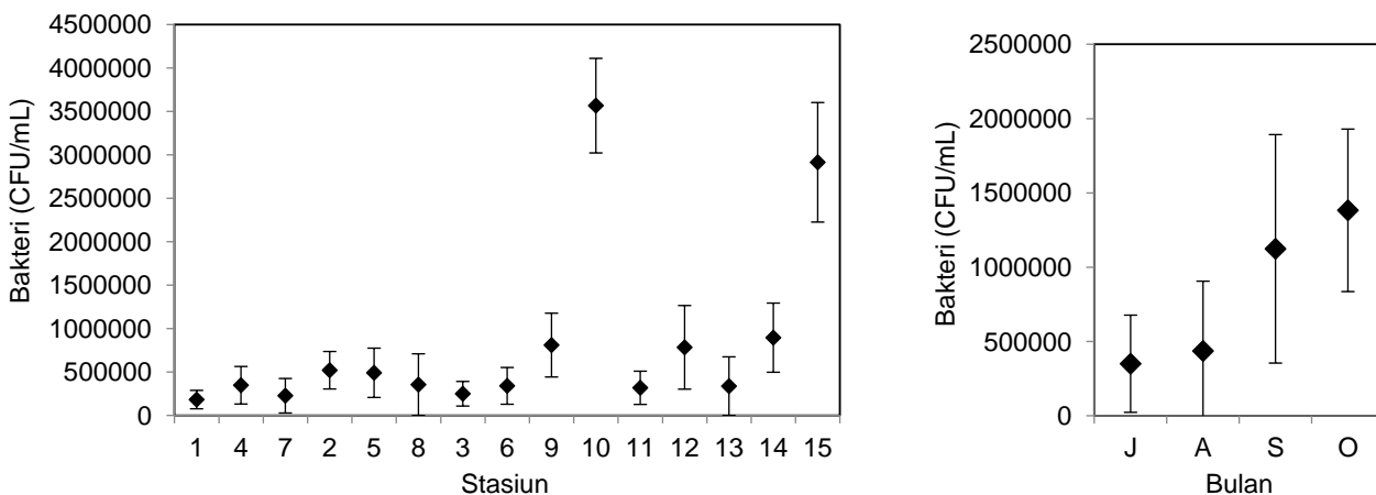
Gambar 2 Spasial dan temporal rerata kelimpahan bakteri heterotrofik di perairan Teluk Jakarta.
