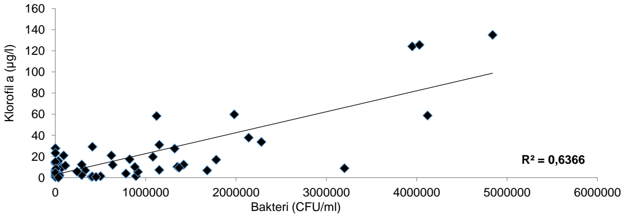
Gambar 5 Scatterplot hubungan kelimpahan bakteri heterotrofik dengan klorofil-a di perairan Teluk Jakarta.
