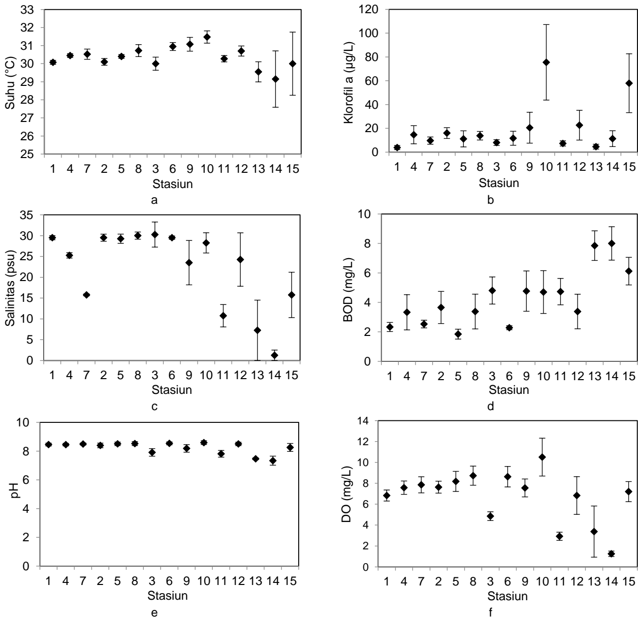
Gambar 3 Rerata suhu (a), klorofil-a (b), salinitas (c), BOD (d), pH (e), dan DO (f) di Perairan Teluk Jakarta.
