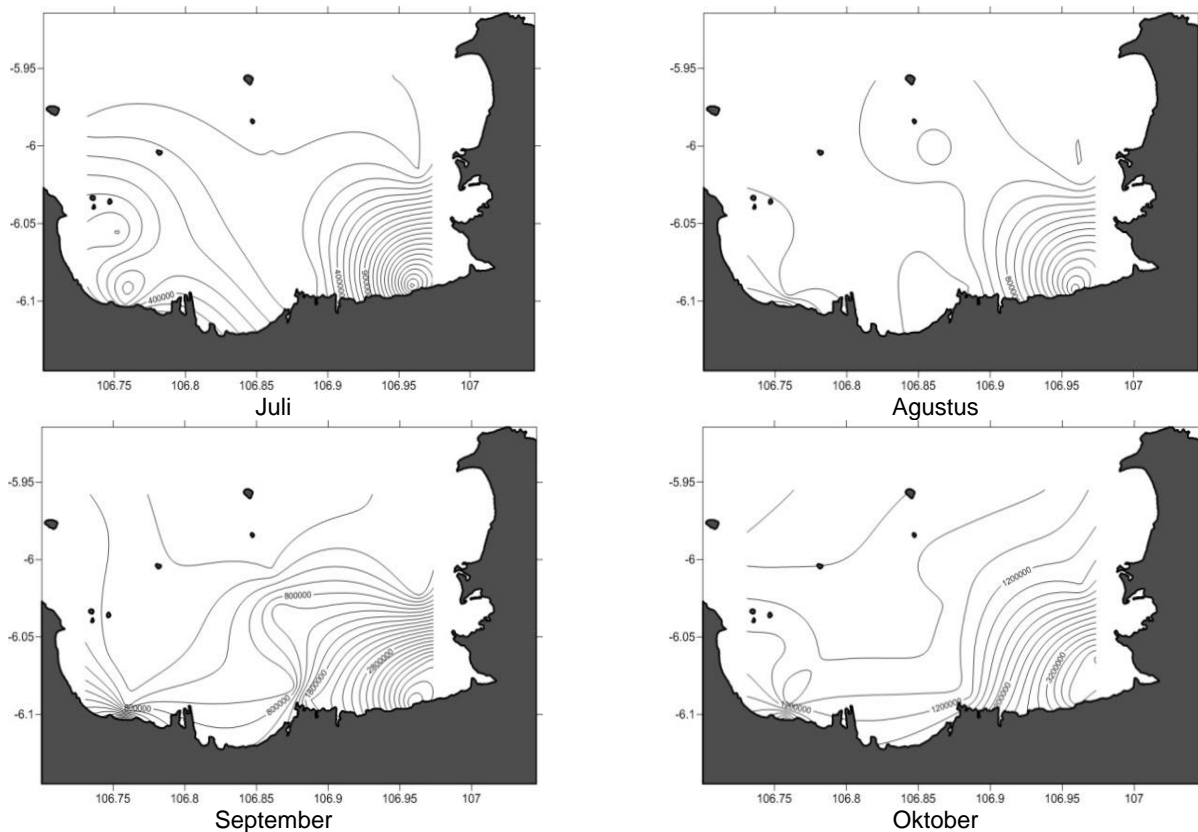
Gambar 4 Pola sebaran horizontal bakteri heterotrofik di perairan Teluk Jakarta.
