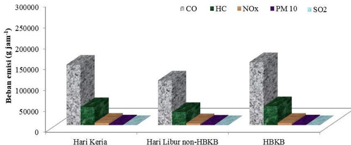
Gambar 3 Perbandingan jumlah polutan CO, HC, NO x , PM 10 , dan SO 2 .
