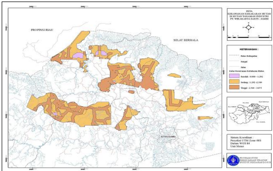
Gambar 5. Peta kerawanan kebakaran hutan di hutan tanaman industri PT. Wirakarya Sakti
