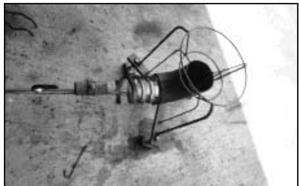
Gambar 3. Kompor bertekanan tipe spiral saat dinyalakan.
