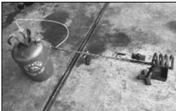
Gambar 2. Kompor bertekanan tipe spiral dengan tabung.
