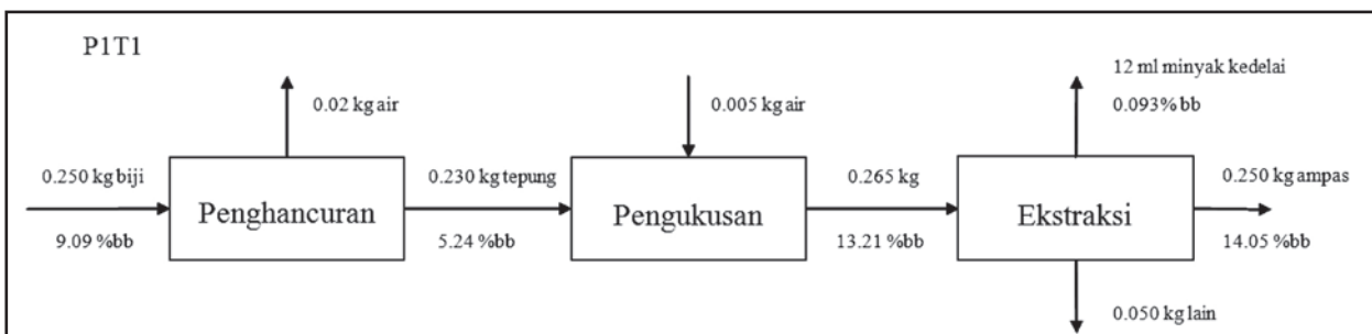
Gambar 5. Keseimbangan massa
