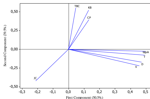
Gambar 1 Hasil analisis PCA pada delapan variabel yang diamati dalam penelitian sengon hasil radiasi sinar gamma
