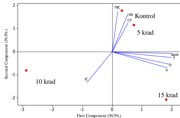
Gambar 2 Hasil analisis BIPLLOT pada delapan variabel yang diamati dalam penelitian sengon hasil radiasi sinar gamma
