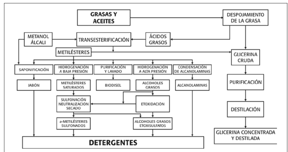
Figura 1. Proceso para la obtención de detergente a partir de grasas y aceites
