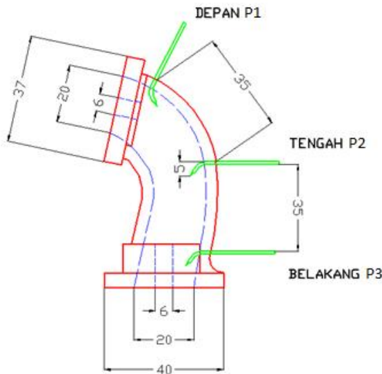
Gambar 3 Posisi penyemprotan ke dalam intake manifold
