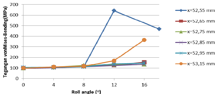
Gambar 3. grafik tegangan vonMises bending yang terjadi pada masing-masing roll angle pada setiap variasi jarak poros.
