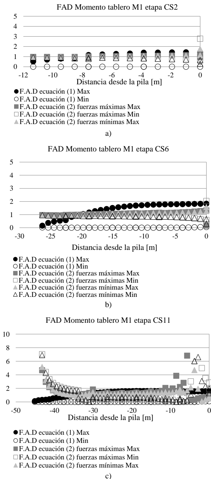
Figura 7. Resultados FAD en la etapa CS2 (a), CS6 (b) y CS11 (c) para el modelo M1 ( H_c/H_p=1 ). Fuente: elaboración propia.
