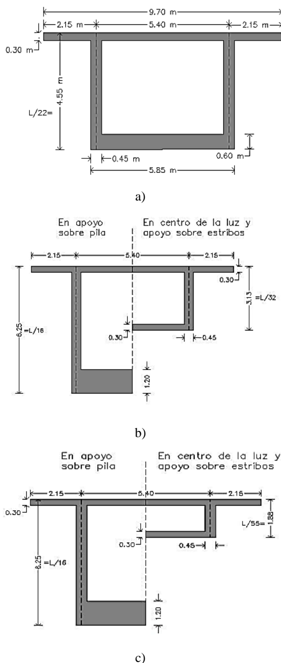
Figura 2. Sección transversal puente viga cajón con sección constante H_c/H_p=1 (a) y sección variable H_c/H_p=0.5 (b) y H_c/H_p=0.3 (c).
