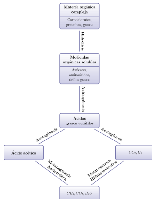
Figura 1. Proceso de digestión anaerobia. Fuente: adaptado de T. Abbasi, S. M. Tauseef, y S. A. Abbasi, Biogas Energy . 2012.
