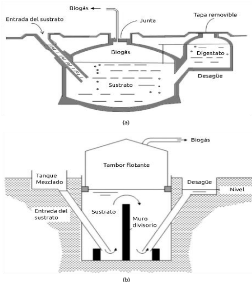
Figura 4. (a) Biodigestor de domo fijo, (b) biodigestor de tambor flotante. Fuente: adaptado de M. Garfí, J. et. al., “Household anaerobic digesters for biogas production in Latin America: A review”.
