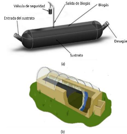
Figura 5. (a) Biodigestor tubular, (b) claustro; adaptación para climas fríos. Fuente: adaptado de M. Garfí, J. et al., “Household anaerobic digesters for biogas production in Latin America: A review”.
