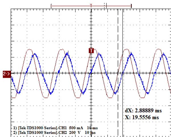
Figura 7. Formas de onda de tensión y corriente para un balasto electromagnético obtenido de la instalación original (año 1968).
