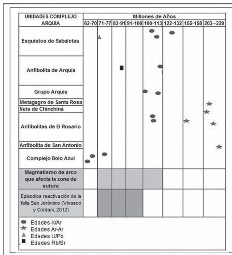
FIGURA 9. Intervalos de edades reportadas para unidades que hacen parte del Complejo Arquía; pulsos magmáticos del arco Cretácico registrados en la zona de convergencia corteza oceánica – corteza continental y episodios de reactivación del sistema de fallas de Romeral en la parte Noroccidental de los Andes según Vinasco y Cordani (2012).
