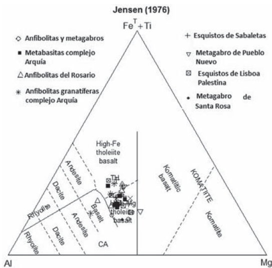
FIGURA 3. Diagrama catiónico Jensen (1976), concentra las muestras del Complejo Arquía en el campo de basaltos toleíticos ricos en Mg.
