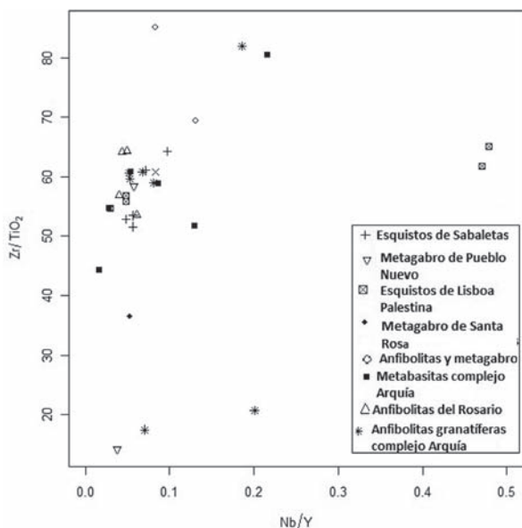
FIGURA 4. Diagrama Zr/TiO 2 vs Nb/Y para las muestras del Complejo Arquía.
