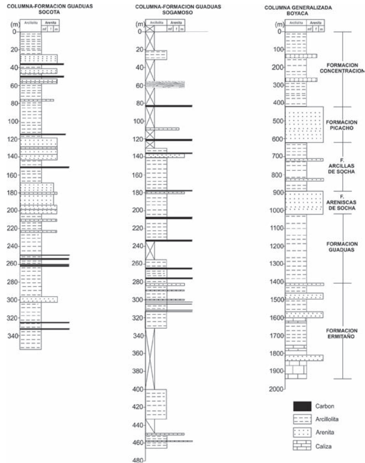
FIGURA 2. A la izquierda, estratigrafía de la Formación Guaduas en Sogomoso y Socotá. A la derecha, estratigrafía regional.
