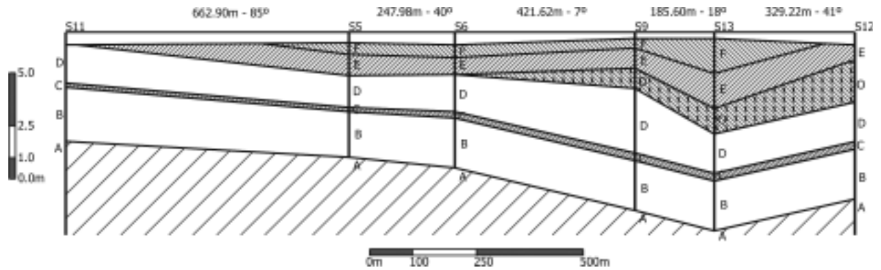
FIGURA 2. Corte geológico del depósito de caolín de la Vereda Barroblanco.
