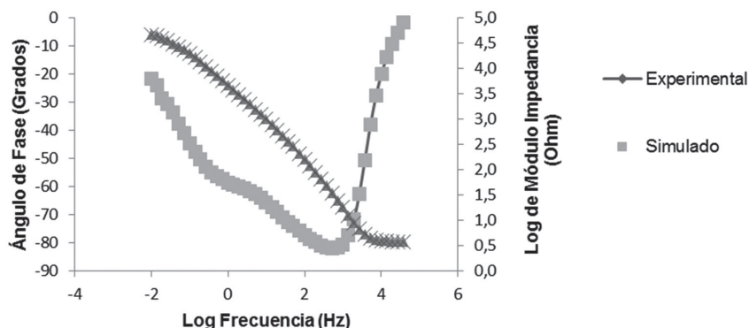
Figura 3. Representación del ajuste de los espectros de Bode mediante simulación en el software Zview.
