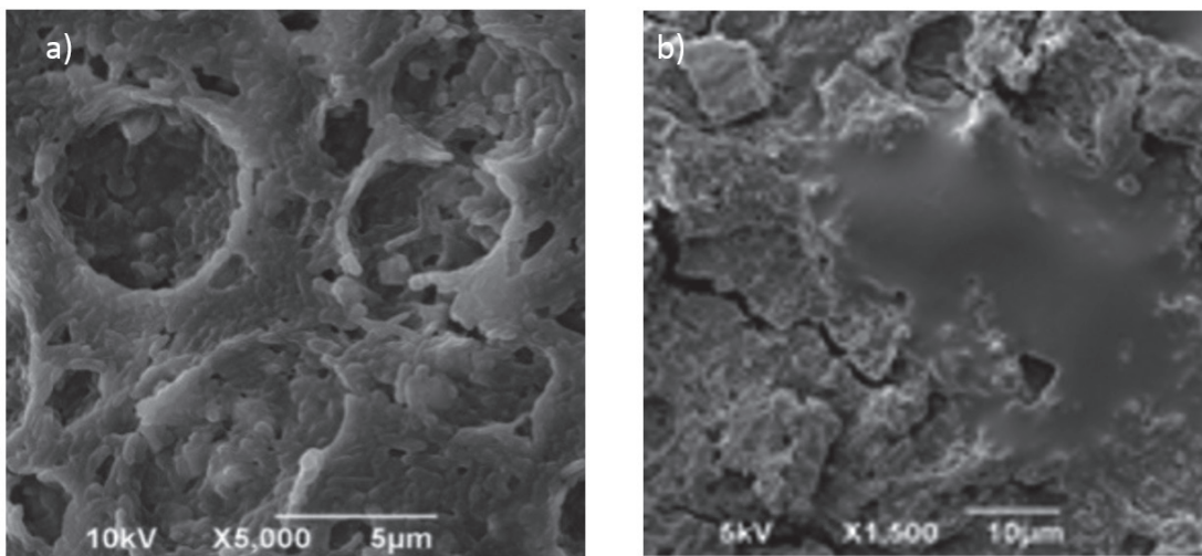
Figura 6. SEM de PLA-PLG-HAP-colágeno, a) sin y b) con células adheridas en su superficie.
