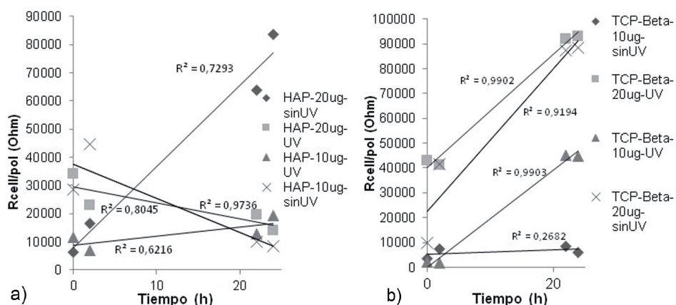
Figura 4. Resistencia a la transferencia de la carga entre las células osteoblásticas y los recubrimientos vs. Tiempo de evolución celular. a) Hidroxiapatita b) fosfato tricálcico β.
