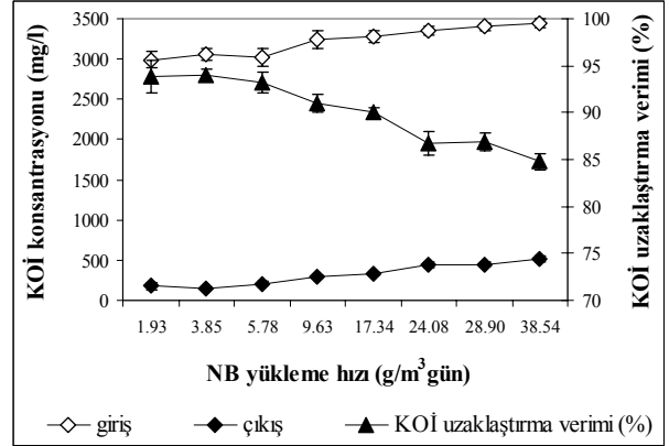
Şekil 2. Artan NB yüklem hızının KOİ uzaklaştırma verimi üzerine etkisi
