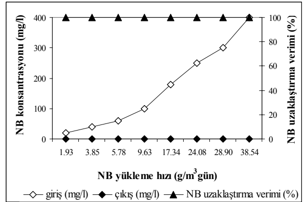
Şekil 3. Artan NB yüklem hızının NB uzaklaştırma verimi üzerine etkisi
