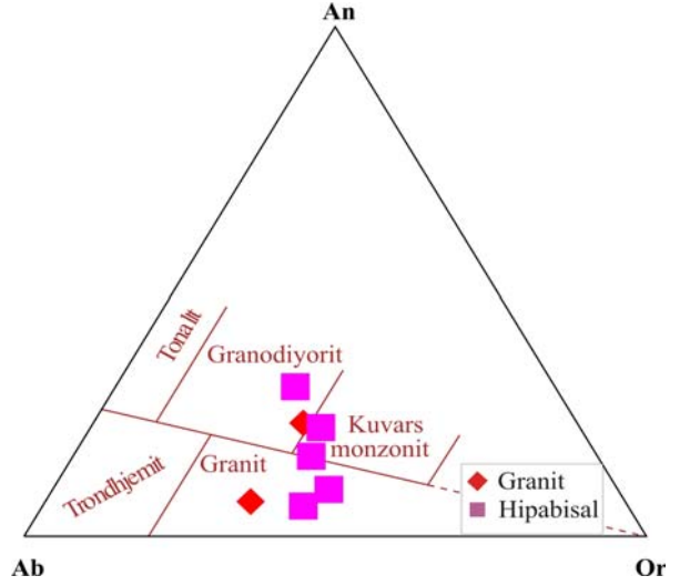
Şekil 7. O'Connor'a(1965) göre CIPW normundan hesaplanan Albit-Anortit- Ortoklaz değerlerine göre granitoyitlerin sınıflandırılması
