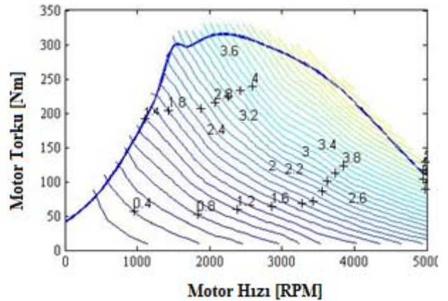
Şekil 11. Yakıt tüketimi
