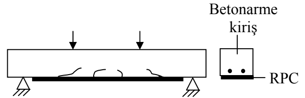
Şekil 9. Çatlamış betonarme kirişin Reaktif Pudra Betonuyla güçlendirilmesi (Karihaloo, 2000; Alae v. diğ., 2001).
