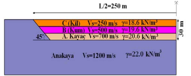
Şekil 2. L=500 m ve H=30 m vadi modeli (M1)
