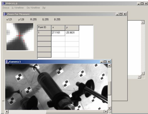
Şekil 4. PMM yazılımı
