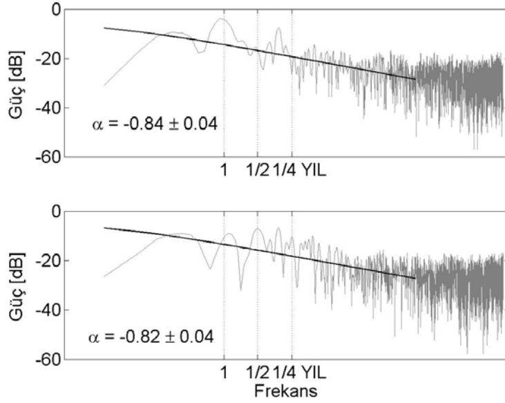
Şekil 5. TRAB zaman serilerinin 1 gün örnekleme aralıklı lineer regresyonu sonrası ölçü düzeltme değerlerinin güç spektrumu
