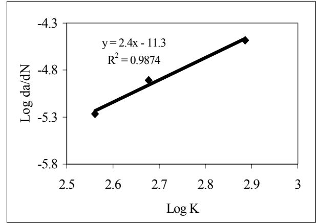
Şekil 14. Kaynaklı bağlantının \log \Delta K_{II} - \log \frac{da}{dN} grafiği
