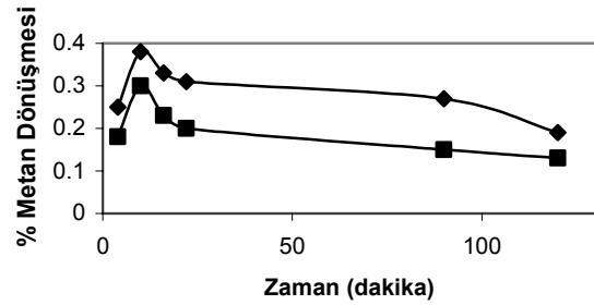
Şekil 5. Düşük metan kısmi basıncında metanın benzene dönüşmesinin zamanla değişimi, reaksiyon şartları: 700°C'de 13 L/saat akış hızında 24:736 CH 4 /Argon gaz karışımı (◆) Dealumine edilmeyen katalizör (■) Okzalik asit ile dealumine edilen katalizör
