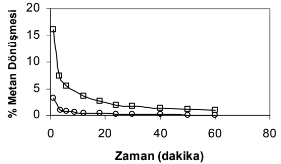
Şekil 11. Metanın hidrokarbon ürünlere dönüşmesinin zamanla değişimi (□) HZSM-5 destekli renyum; (○) CaZSM-5 destekli renyum
