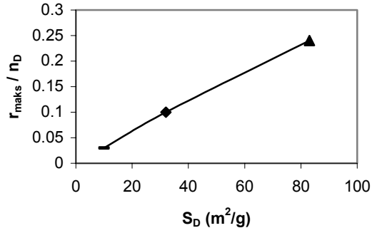
Şekil 10. Zeolit dış yüzeyinde bulunan birim asit merkez başına düşen maksimum hidrokarbon oluşum hızının dış yüzey alanı ile değişimi (◆) Si/Al=14 ; (▲) Si/Al=28 ; (—) Si/Al=54
