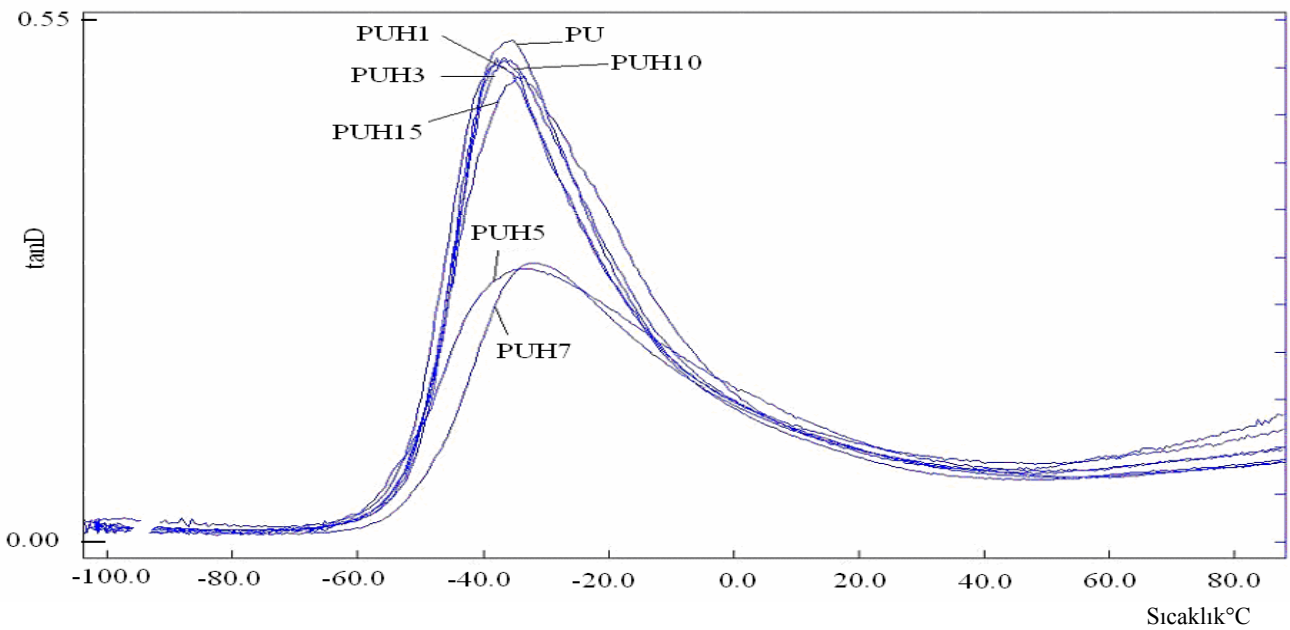
Şekil 8. PU ve nanokompozitlerinin tan delta değerleri
