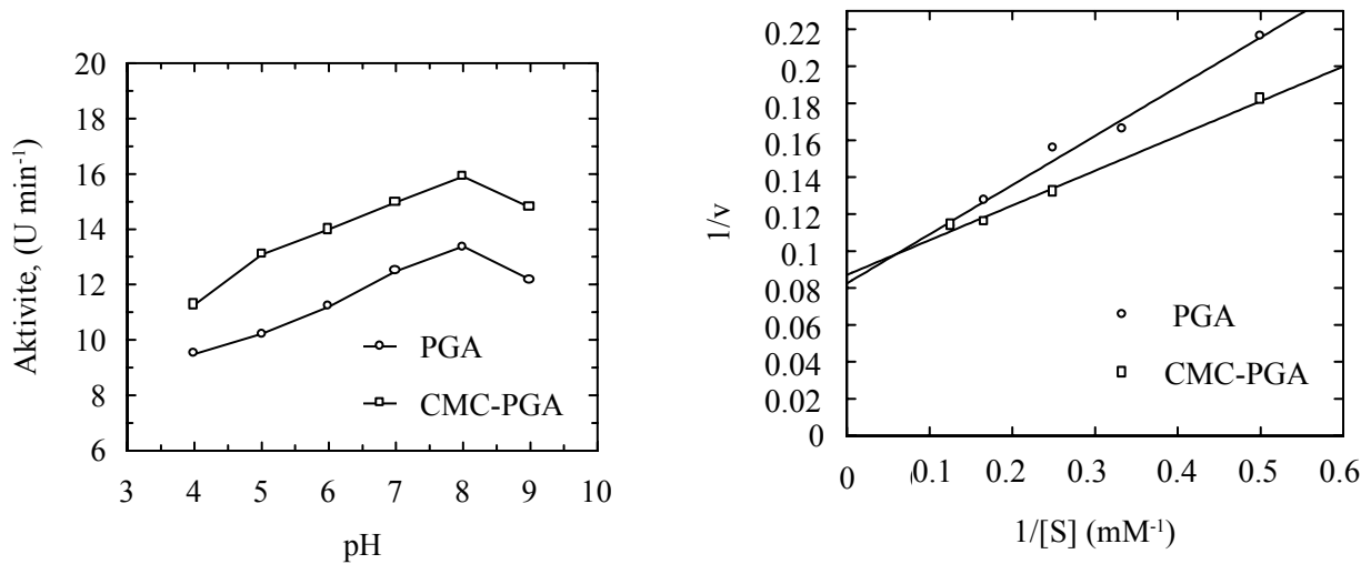
Şekil 3. PGA ve CMC-PGA için çizilen Lineweaver-Burk diyagramı (nativ PGA ve CMC-PGA için r değerleri sırasıyla 0.9935 ve 0.9963'tür).
