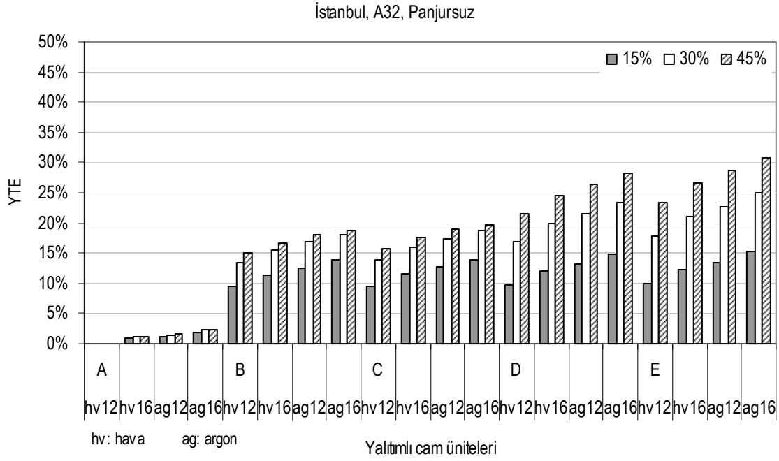
Şekil 2. Panjursuz YCÜ'lerin 6/12/6mm hava dolgulu berrak çift cama göre toplam enerji kullanımında sağladığı azalma miktarı (%)
