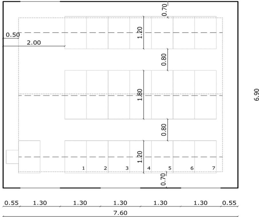
Şekil 6. Derslik planı
