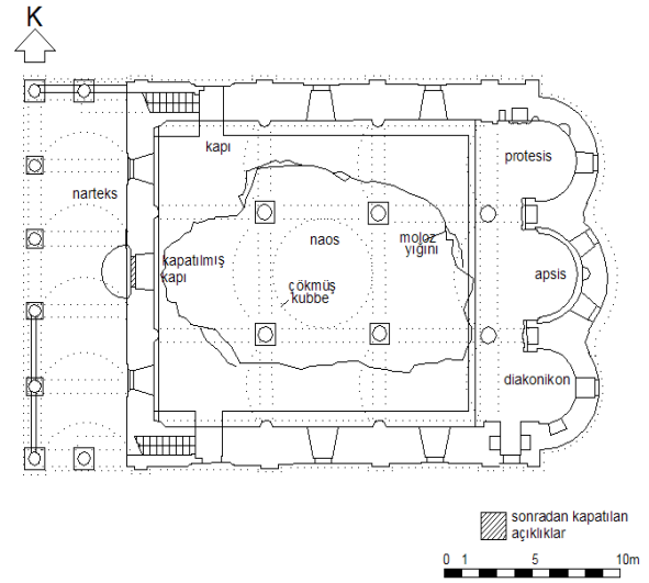
Şekil 6. Yanartaş Manastır Kilisesi zemin kat planı (Ş. Güngör Açıkgöz)
