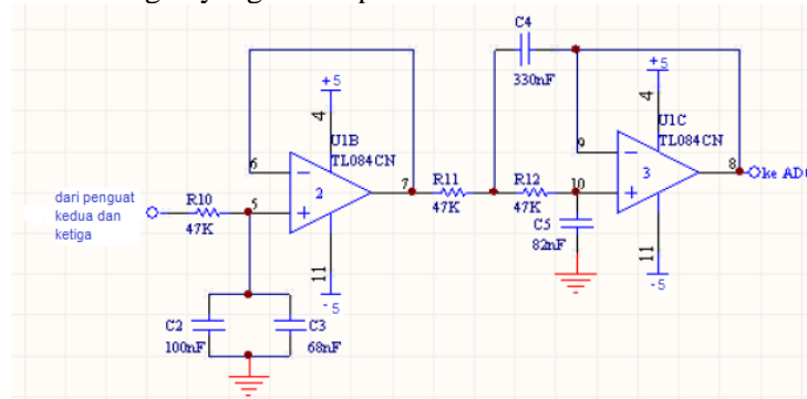
Gambar 13. Realisasi LPF yang digunakan
