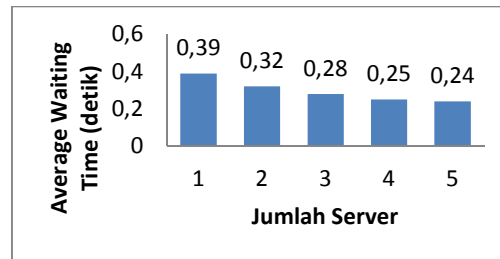
Gambar 9. Grafik Average Waiting Time Penambahan Jumlah Server
