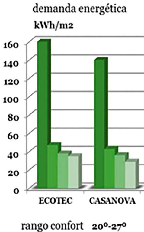
Figura 4. Tabla comparativa de demandas energéticas según premisas de cálculo con ECOTECT y CASANOVA sobre 4 tipos de proyecto
