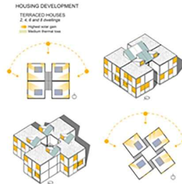
Figura 5. Algunos esquemas de agrupamiento en la parcela de la vivienda CASA+
