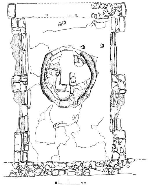
Fig. 12.—Planta general de la nave central del baptisterio con la cuarta piscina.
