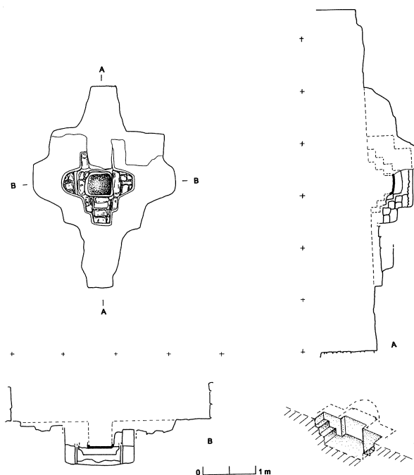
Fig. 10.—Planta de la tercera piscina, con secciones longitudinales este-oeste (A) y norte-sur (B) y esquema reconstructivo.
