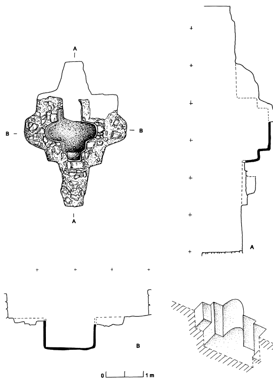
Fig. 6.—Planta de la primera piscina, con secciones longitudinales este-oeste (A) y norte-sur (B) y esquema reconstructivo.
