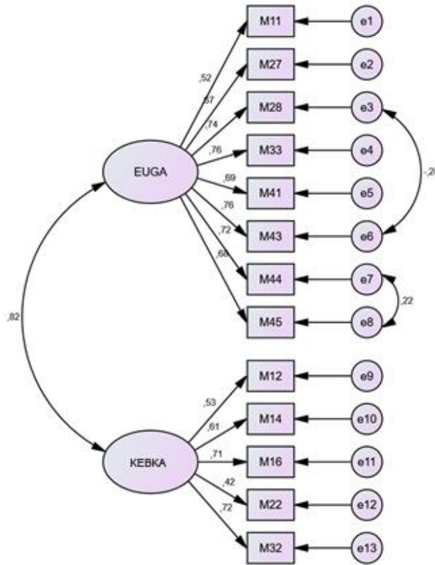
Şekil 1. TCEÖ doğrulayıcı faktör analizi modeli (standartlaştırılmış değerler).
