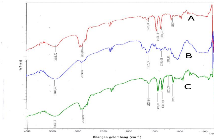
Gambar 1. Spektrum FTIR (A) polipropilena, (B) biomassa alang-alang, dan (C) biokomposit alang-alang dengan polipropilena.
